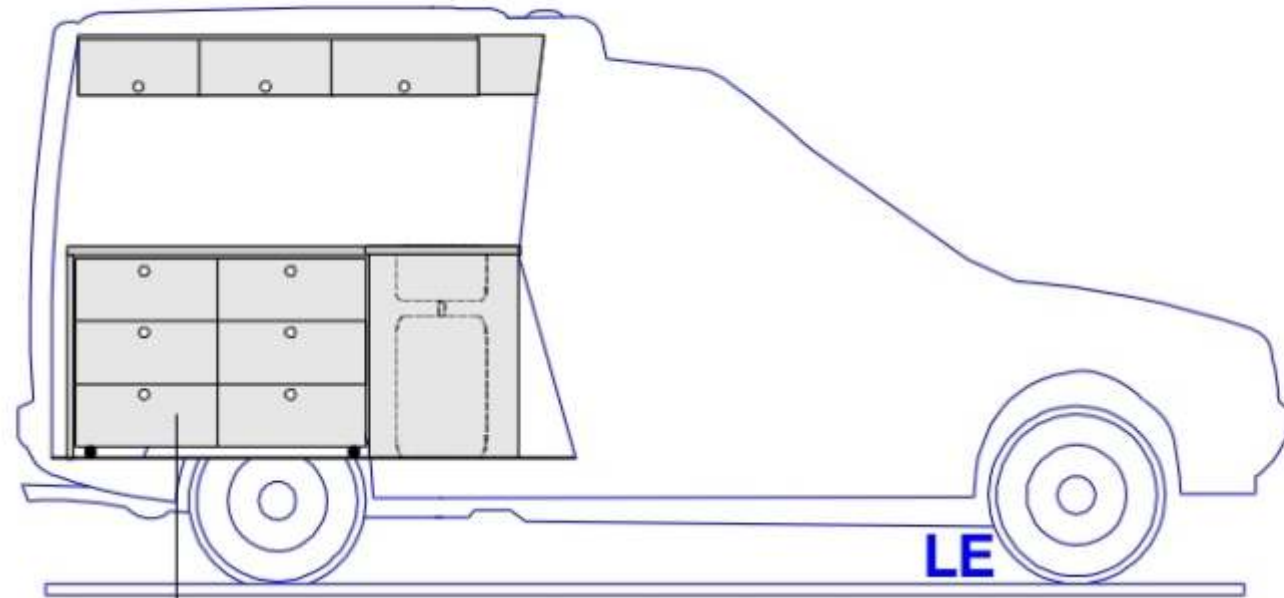
TEIRO MÓVEL X 960L X 620A TAS C/ DIVISÃO TIPO COLMEIA IDAS DEFINIR NA MONTAGEM )
